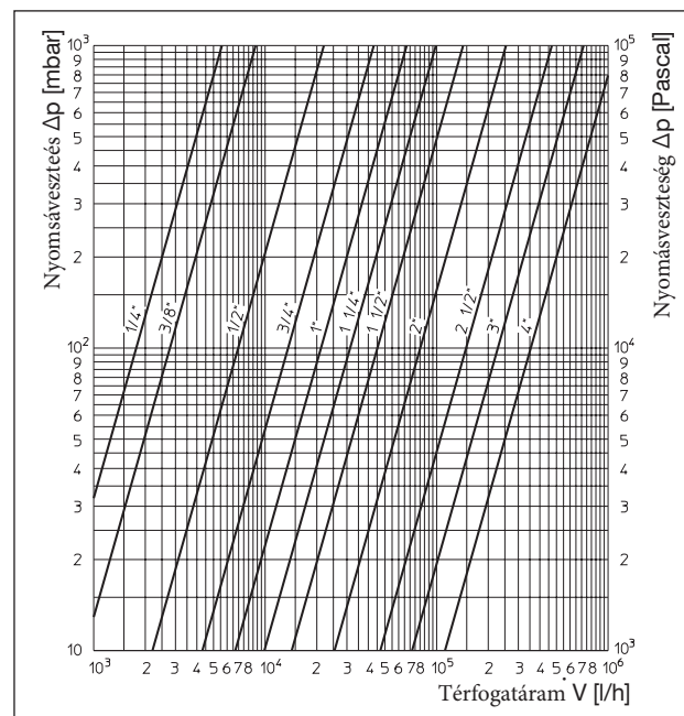
Átfolyási diagram
