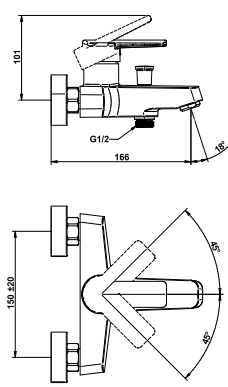
Kádtöltő csaptelep
