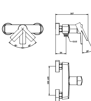
Zuhany csaptelep
