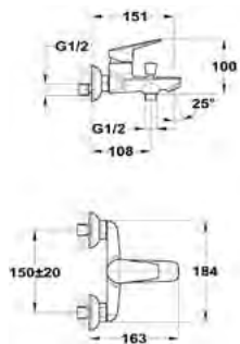
Kádtöltő csaptelep
