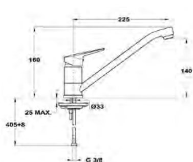
Mosogató csaptelep
