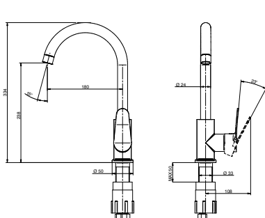
Mosogató csaptelep
