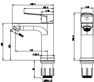
Mosdó csaptelep
