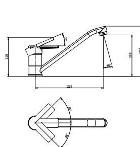
Mosogató csaptelep
