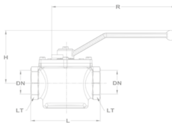
Gömbcsap BB menettel
