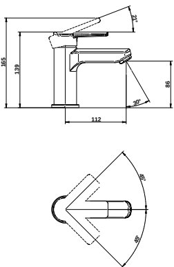
Mosdó csaptelep
