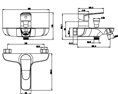
Kádtöltő csaptelep
