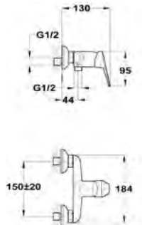
Zuhany csaptelep
