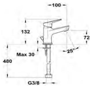
Mosdó csaptelep
